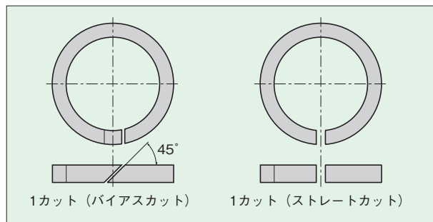
図2 分割方式
