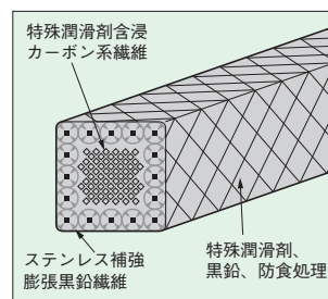
図3 TOMBO No.2250-Aの断面図
