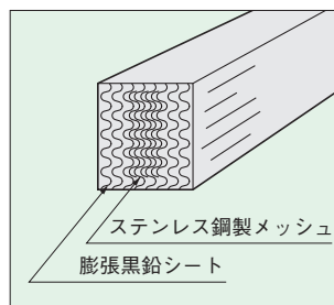
図1 TOMBO No. 2205の断面図
