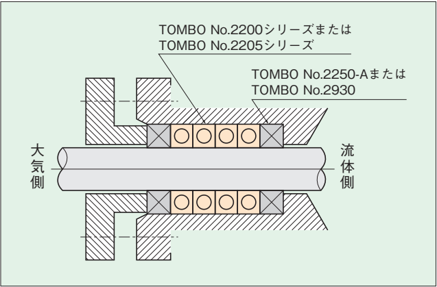
図4 高温バルブ用パッキンの組み合わせ方
