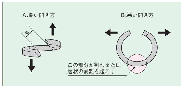
図5 装着要領
