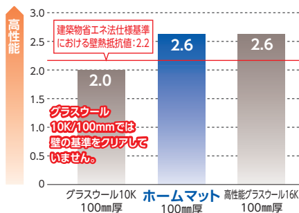
断熱材別 熱抵抗値の比較
